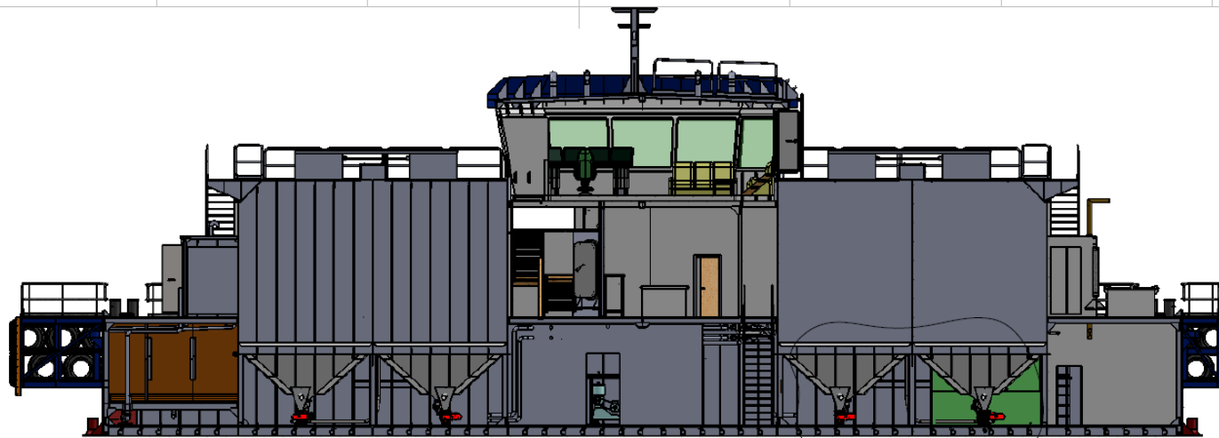
SECTION D-D SCALE 1 : 125
