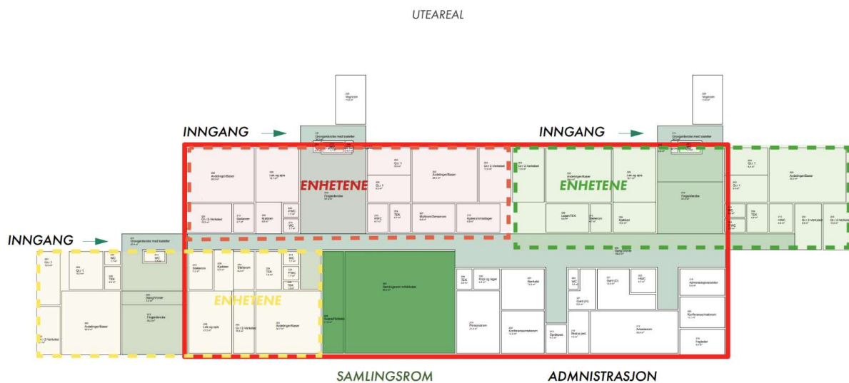
Figur 22: Plantegning konsept 1
