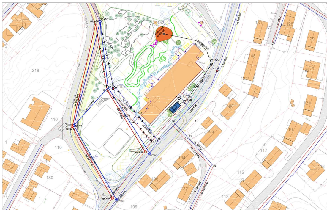
Figur 31: VA-anlegg
