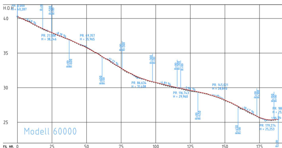
Figur 35: Fall på gang- og sykkelveg følger Idrettsvegen
