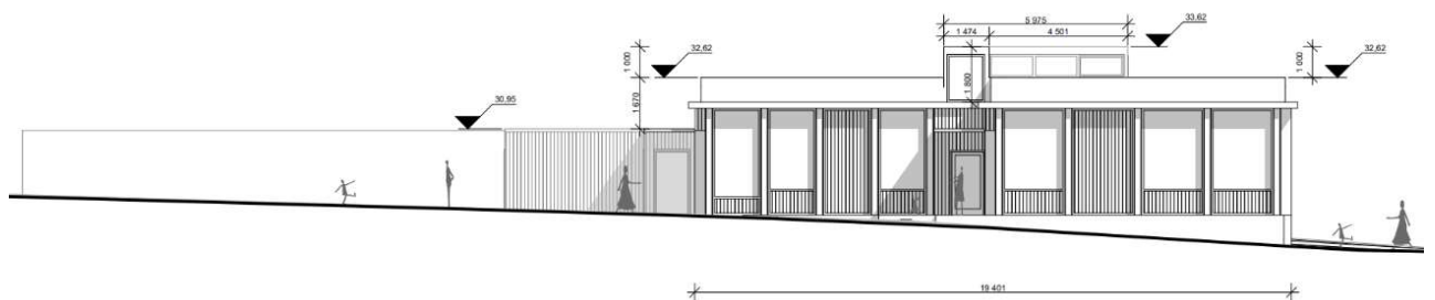
Figur 26: Fasade mot sør/Idrettsvegen
