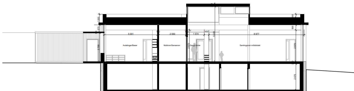
Figur 43: Typisk snitt gjennom bygget øst-vest
