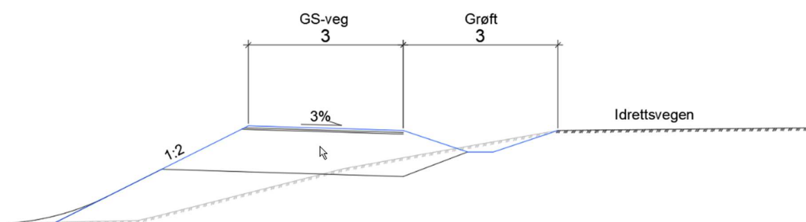
Figur 34: Tverrsnitt av gang- og sykkelveg
