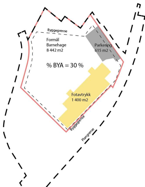
Figur 30: Planlagt utnyttelse innenfor bebyggelsesformål; barnehage
