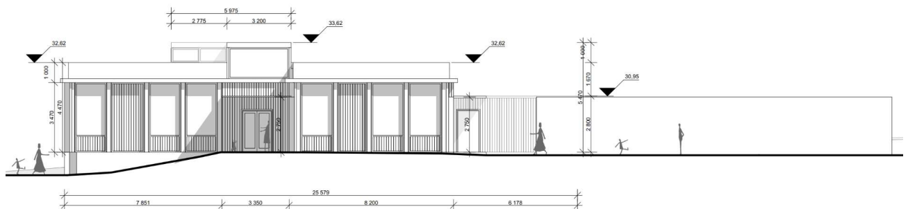
Figur 27: Fasade mot nord
