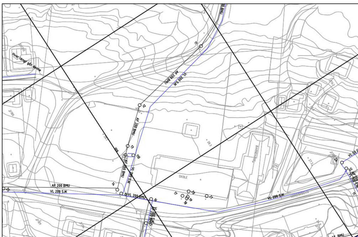
Figur 18: Ledningskart VA eksisterende situasjon.
